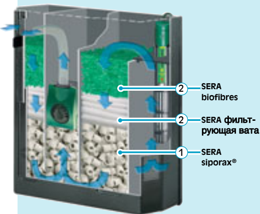
SERA внутренний биофильтр В
