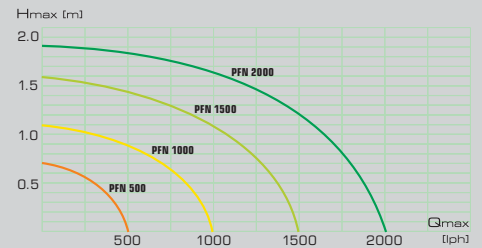
Соотношение производительности помпы и максимальной высоты подъема воды Débit de la pompe par rapport à l'hauteur de levage de l'eau
